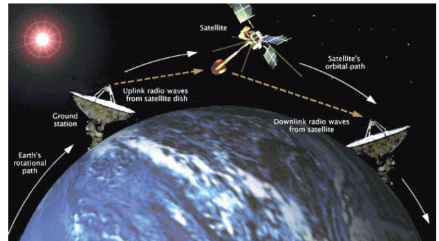
ภาพที่ ๑ ภาพสถานีรับ - ส่ง ดาวเทียม
