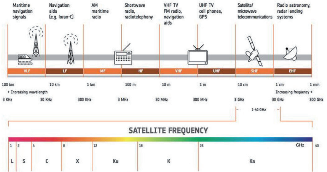
ภาพที่ ๗ แผนภาพแสดงย่านความถี่ที่ถูกนำมาใช้งานสำหรับกิจการอวกาศ โดยการใช้ตัวอักษรกำกับเพื่อให้ง่ายต่อการอ้างถึงมากกว่าการใช้ตัวเลข
